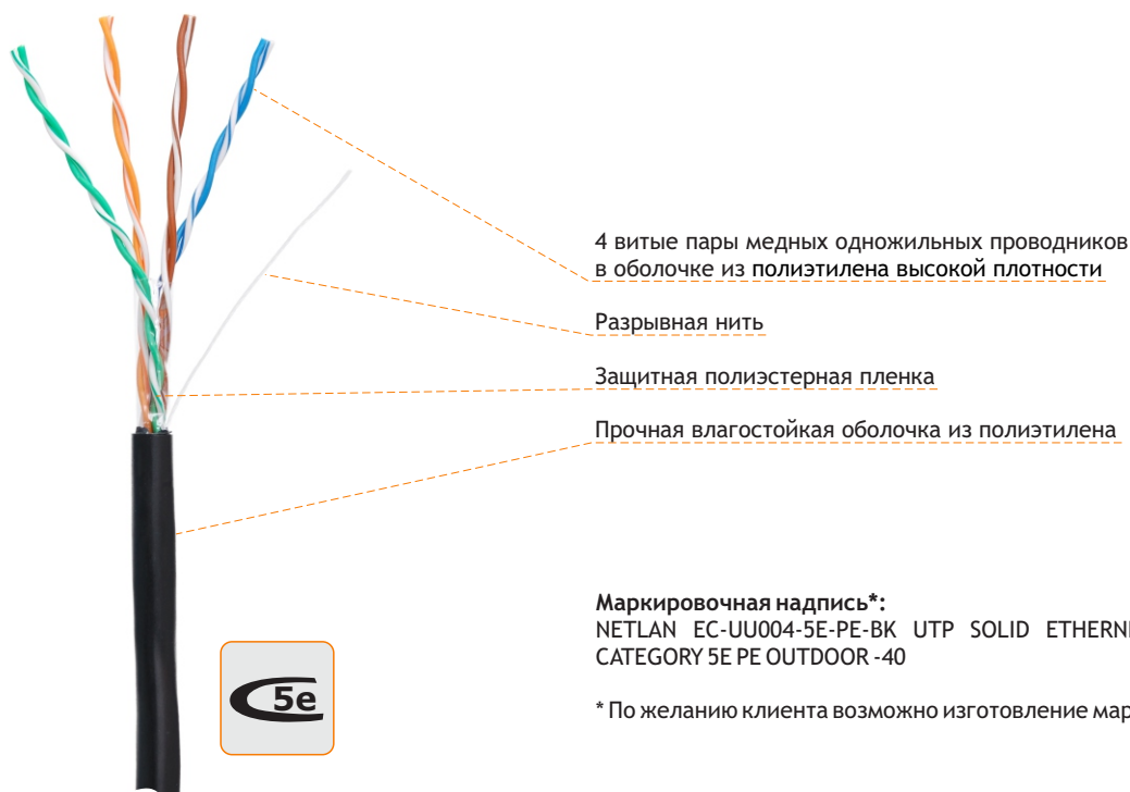
ЕС-UU004-5E-PE-BK-1
